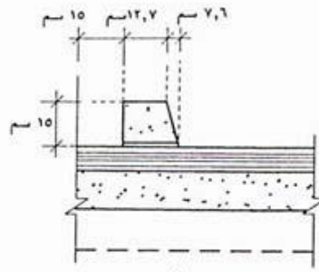
مصدة مثبتة بالأرضية بمادة الايوكسي اللاصقة
