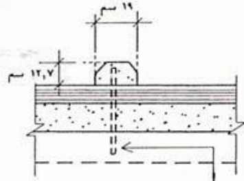
قضبان من حديد تسليح مغروسان عمودياً لتثبيت المصدة بالأرض (البعد ١٢.٧ و ١٩)
